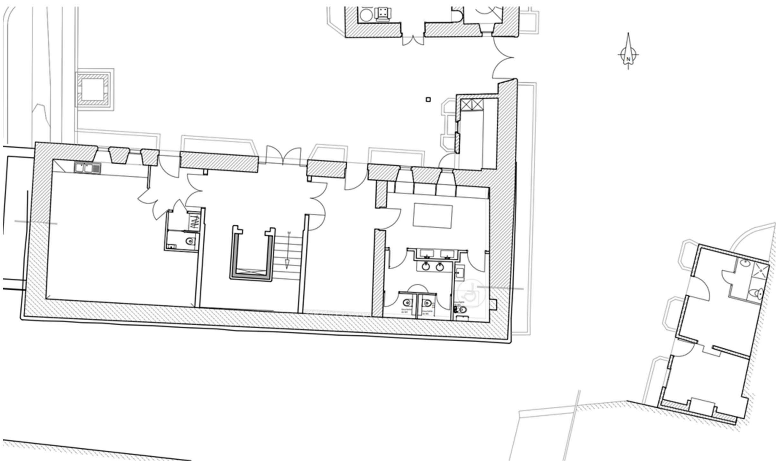
Plan RDC - PETIT LOGIS
