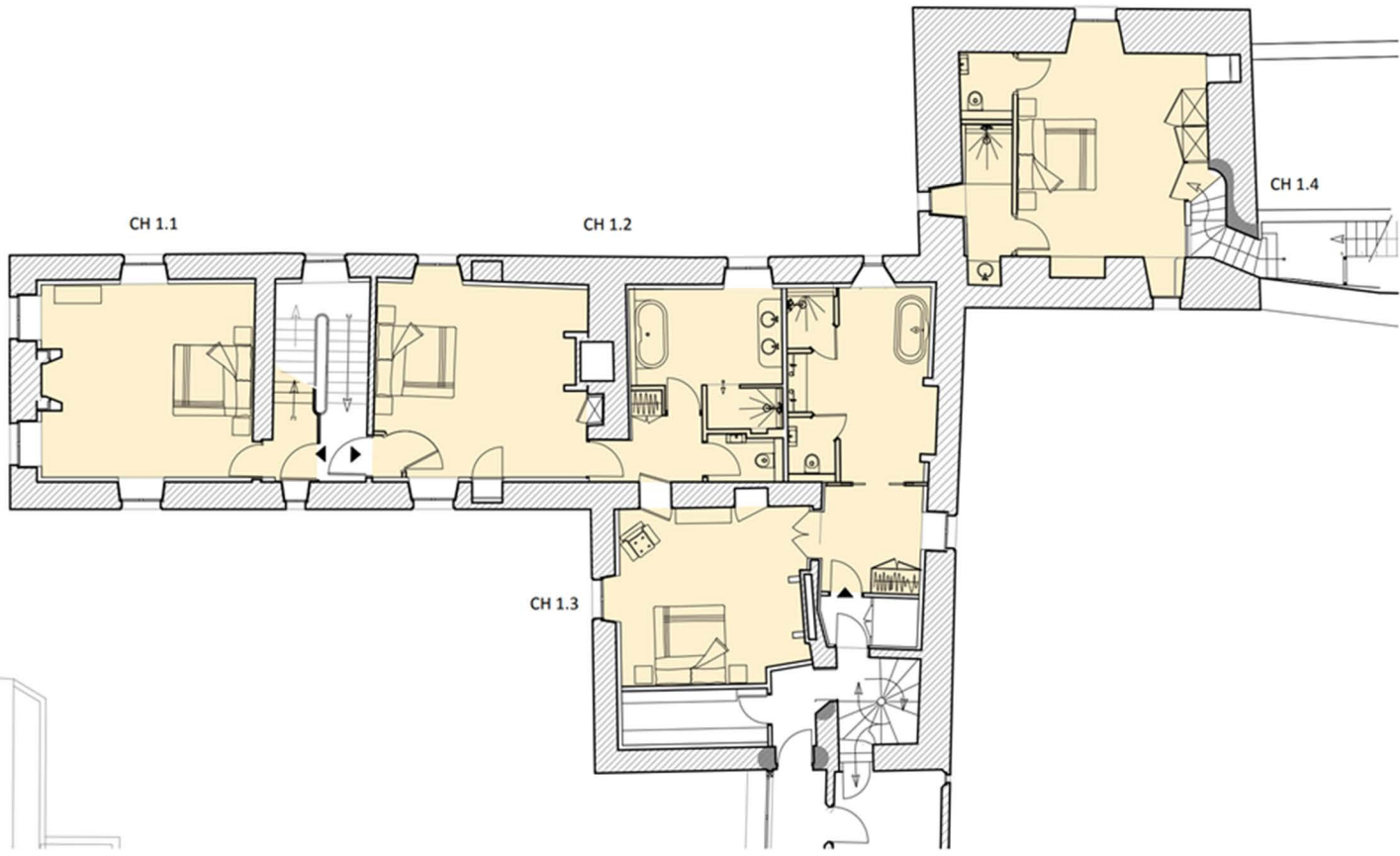
Plan étage - GRAND LOGIS
